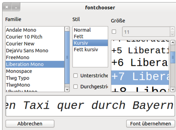
Abbildung 23.2.0.1: Font-Chooser
